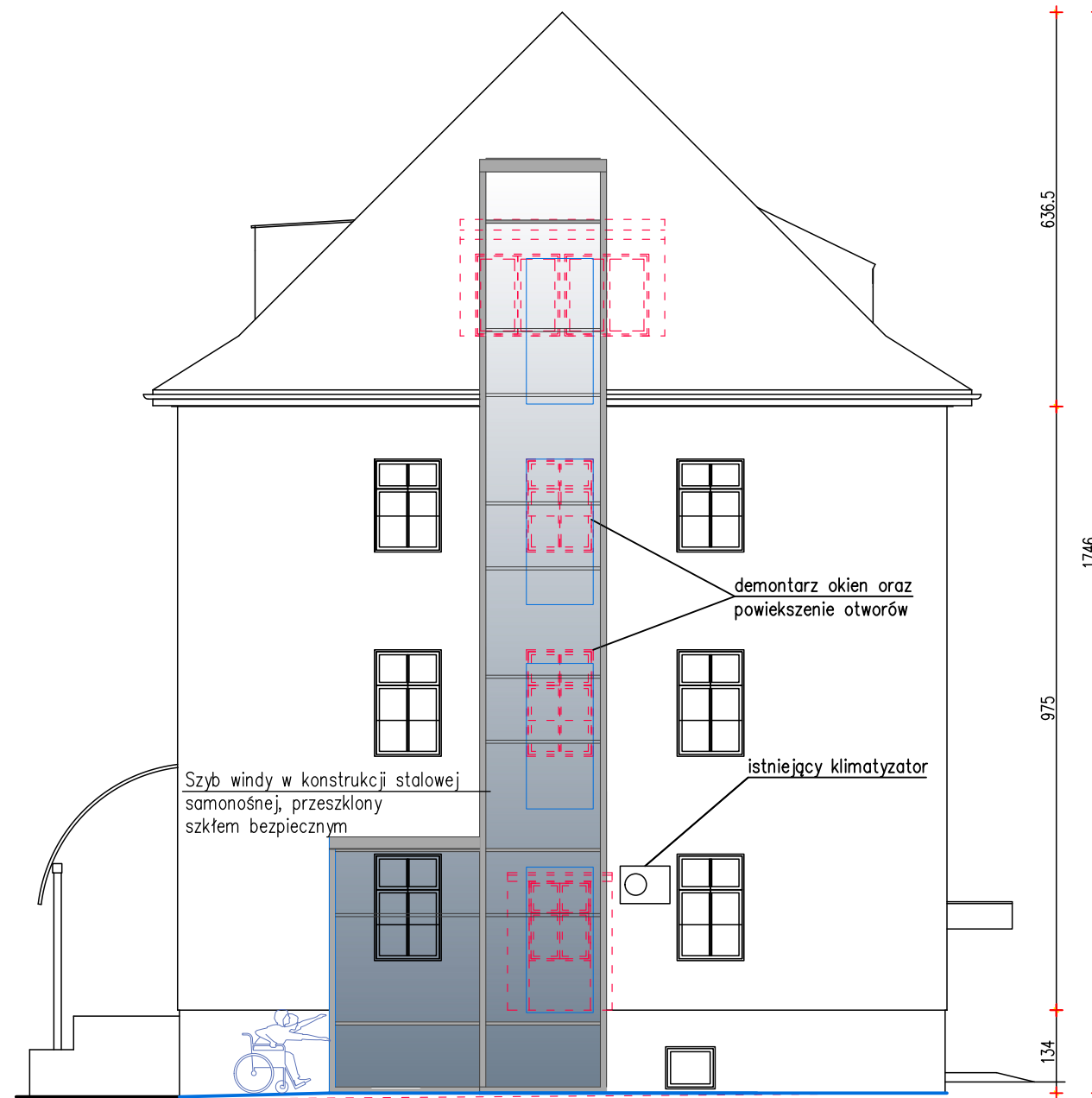
ELEWACJA WSCHODNIA
