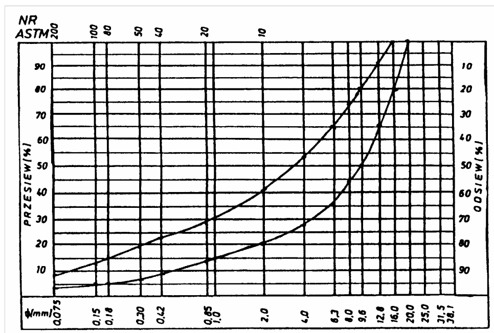
Krzywe graniczne dla mieszanki 0-20mm na wyrównanie podbudowy KR-2
