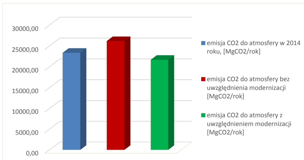
Wykres 17 Emisja CO 2 do atmosfery w 2014 roku i prognoza na 2020 rok na terenie gminy Żarnów w sektorze mieszkaniowym
