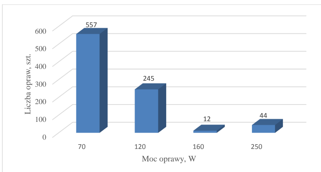
Wykres 8. Podział oświetlenia ulicznego w gminie Żarnów
