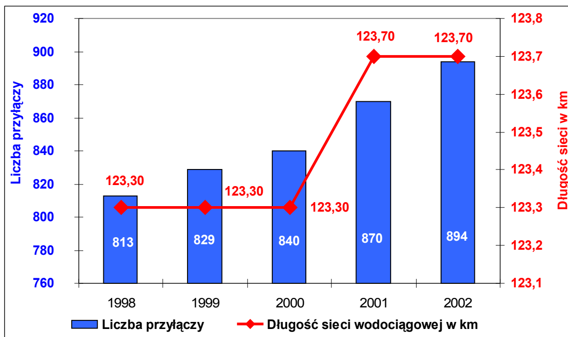
Wykres 7.2. Długość sieci wodociągowej i liczba przyłączy w Gminie w latach 1998-2002
